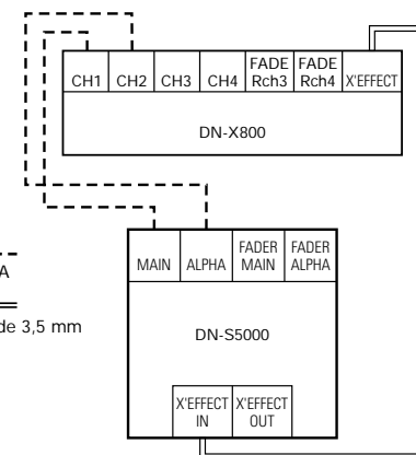
Fig.2: Conexiones X-Effect ejemplo 1
